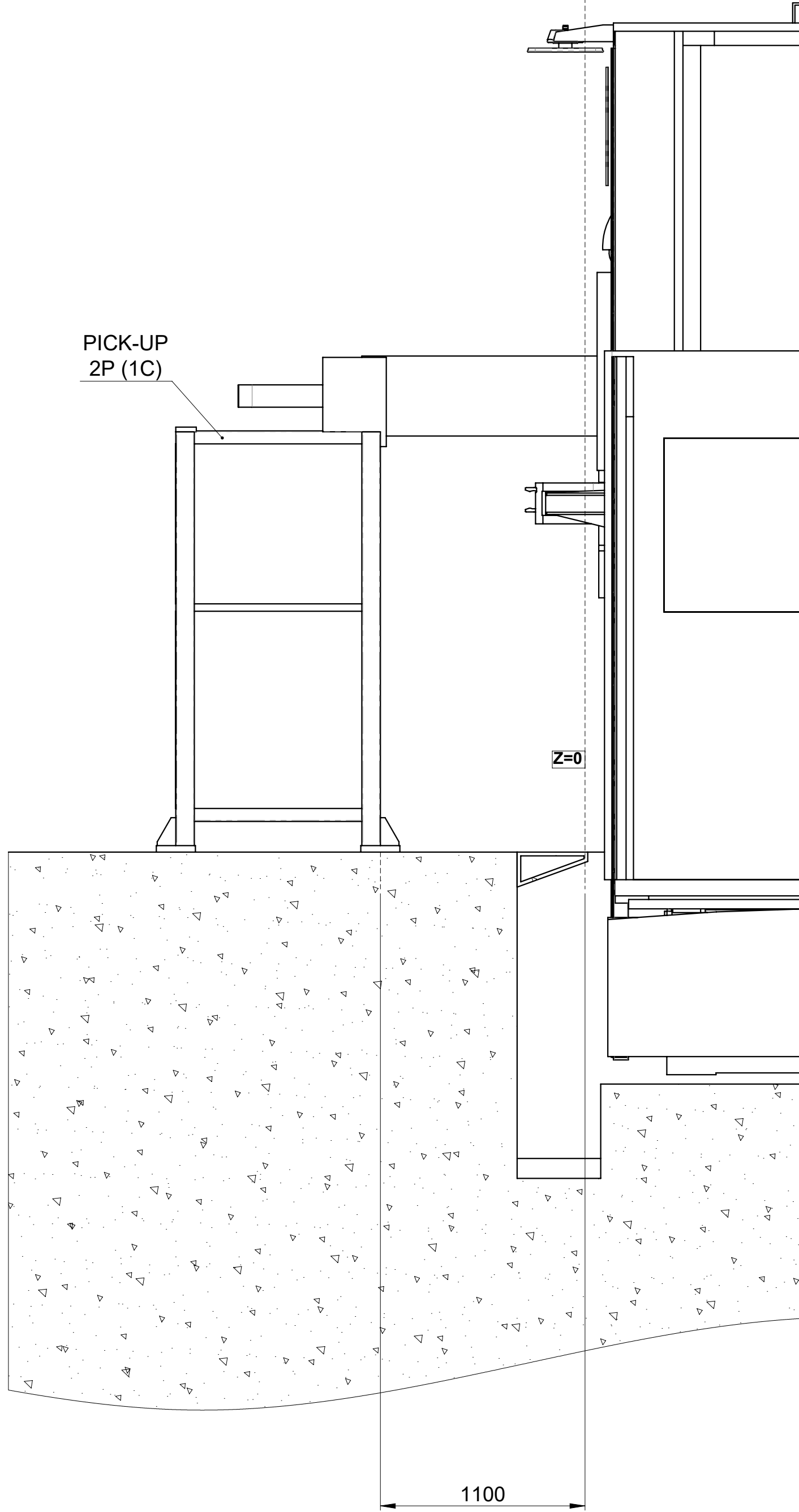
A-A 270°
